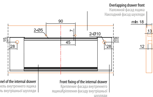
Overlapping drawer front Наложной фасад ящика Накладний фасад шухляди
