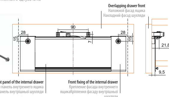
Front fixing of the internal drawer Крепление фасада внутреннего ящика Кріплення фасаду внутрішньої шухляди
